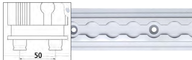
GSP-System für Airlineschiene mit 25 mm Raster
