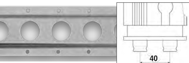
GSP Getränkeperrbalken System für Rundloch-Ankerschielen mit 40 mm Raster
