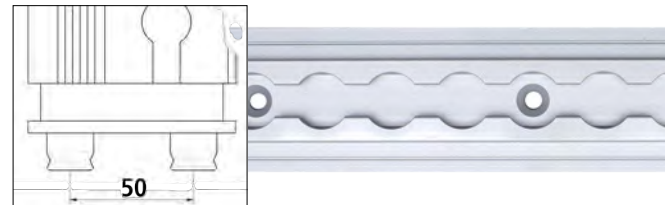
GSP-System für Airlineschielen mit 25 mm Raster
