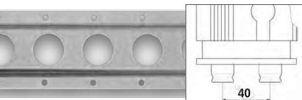
GSP Getränkeperrbalken System für Rundloch-Ankerschiene mit 40 mm Raster
