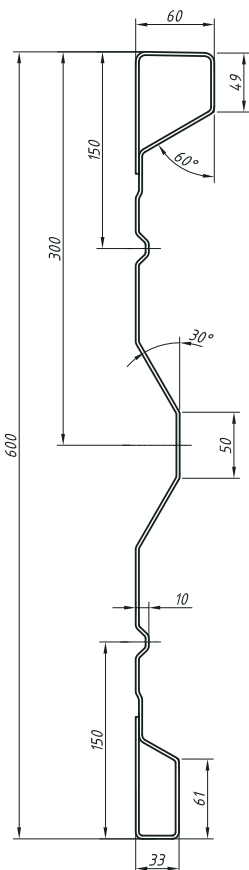
Rysunek SU-600/60/33
