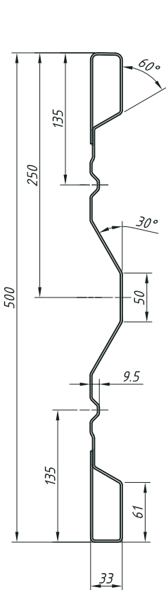
Rysunek SU-500/33/33
