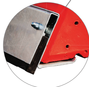
Wypożenie specjalne „SOFT TOUCH” dodatkowo z blachą zaciskową 4 mm i gumą 2200 x 258 x 30 mm
